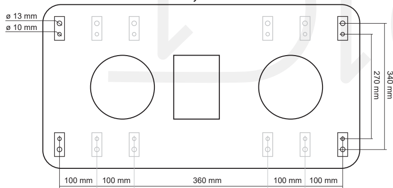
Půdorys kotvení
