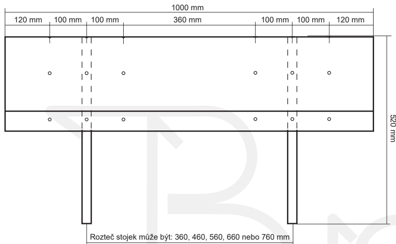
Půdorys kotvení
